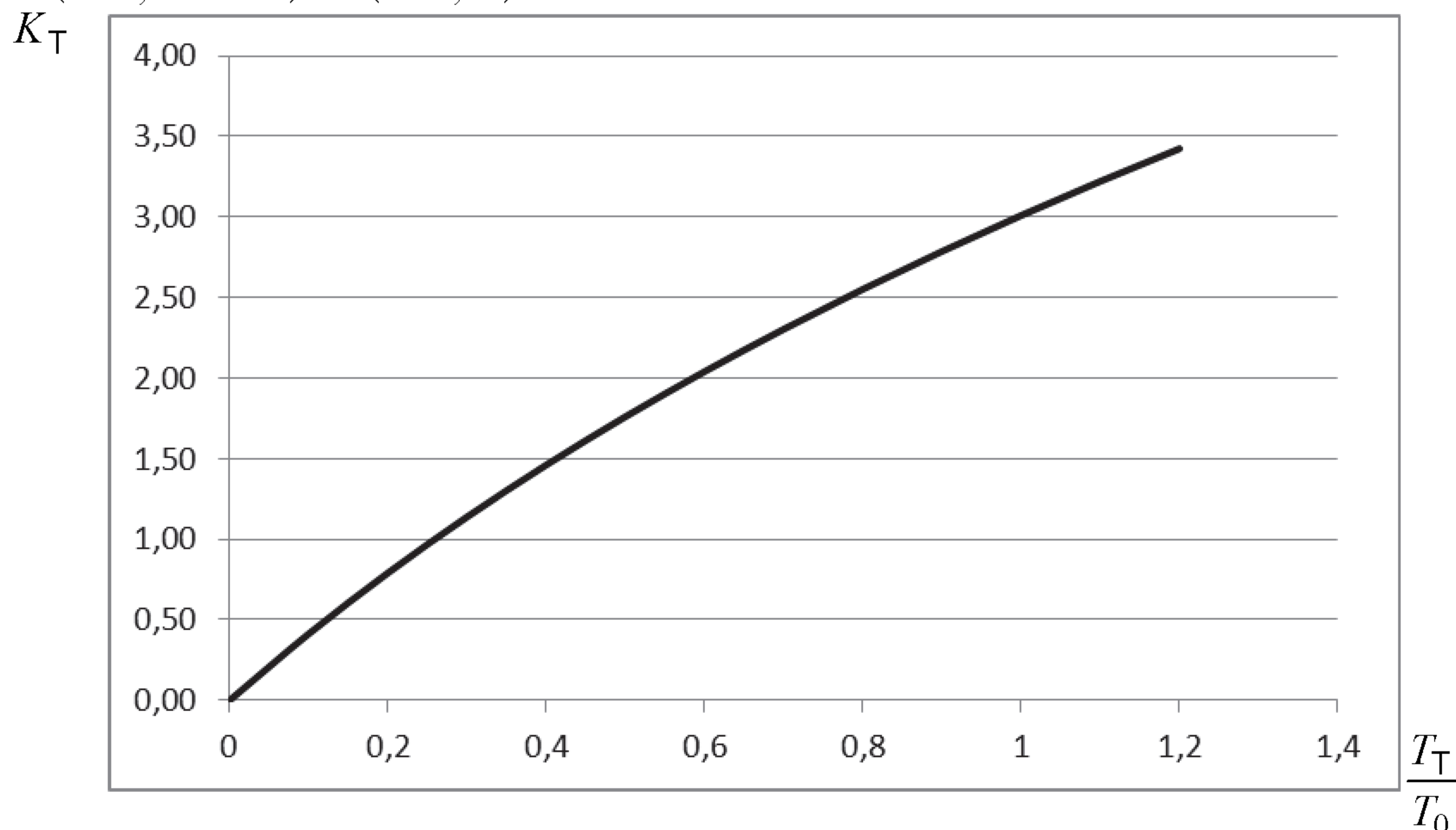
Рисунок А.1 – Зависимость K_T , дБ, от T_T/T_0
